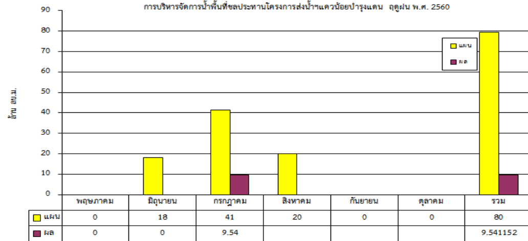
การบริหารจัดการน้ำพื้นที่ชลประทานโครงการส่งน้ำแควน้อยบำรุงแดน ฤดูฝน พ.ศ. 2560
