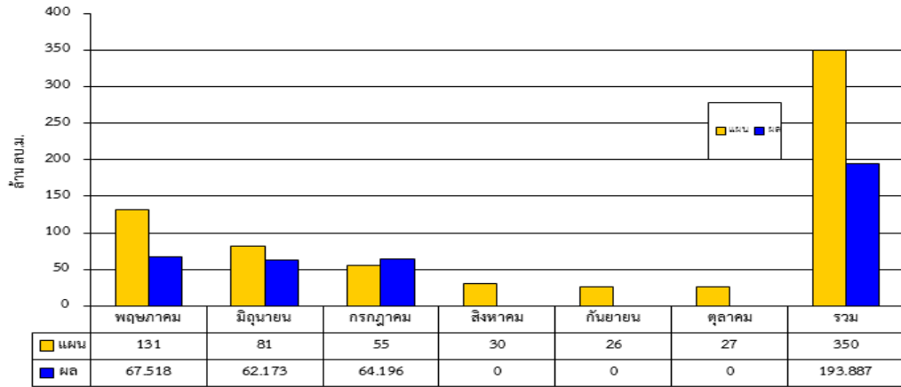
การบริหารจัดการน้ำเขื่อนแควน้อยบำรุงแดนฤดูฝน พ.ศ. 2560
